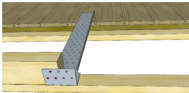
Figuur 3 - Sparring op hart voorzijde overstekbeugel
