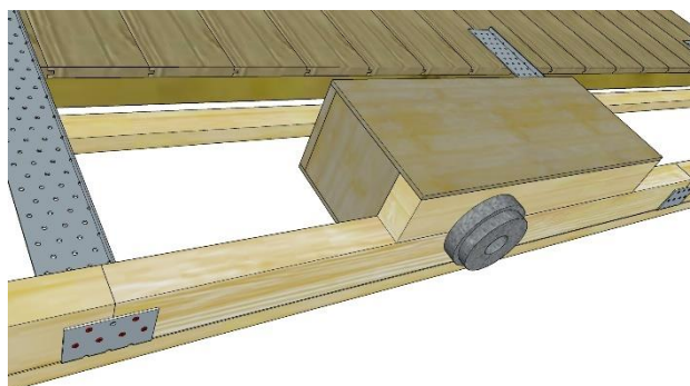
Figuur 4 - Gemonteerde Uni-Nestkast
