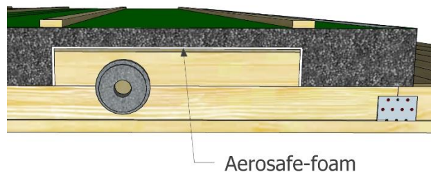
Figuur 9 - Aerosafe-foam
